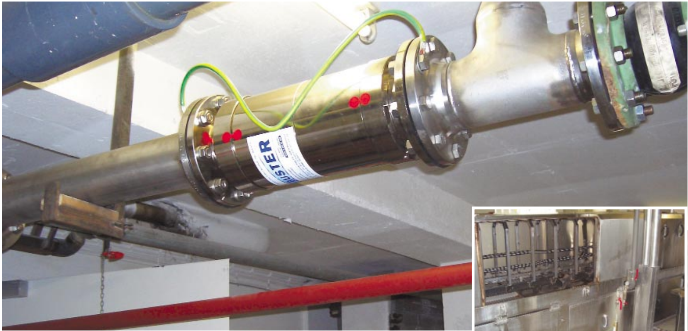
Die Größe des Scale Busters wird in Abhängigkeit von Volumenstrom des Wassers ausgewählt, die Installation erfolgt direkt in die Zuleitung. Fotos: ISB Watertec
